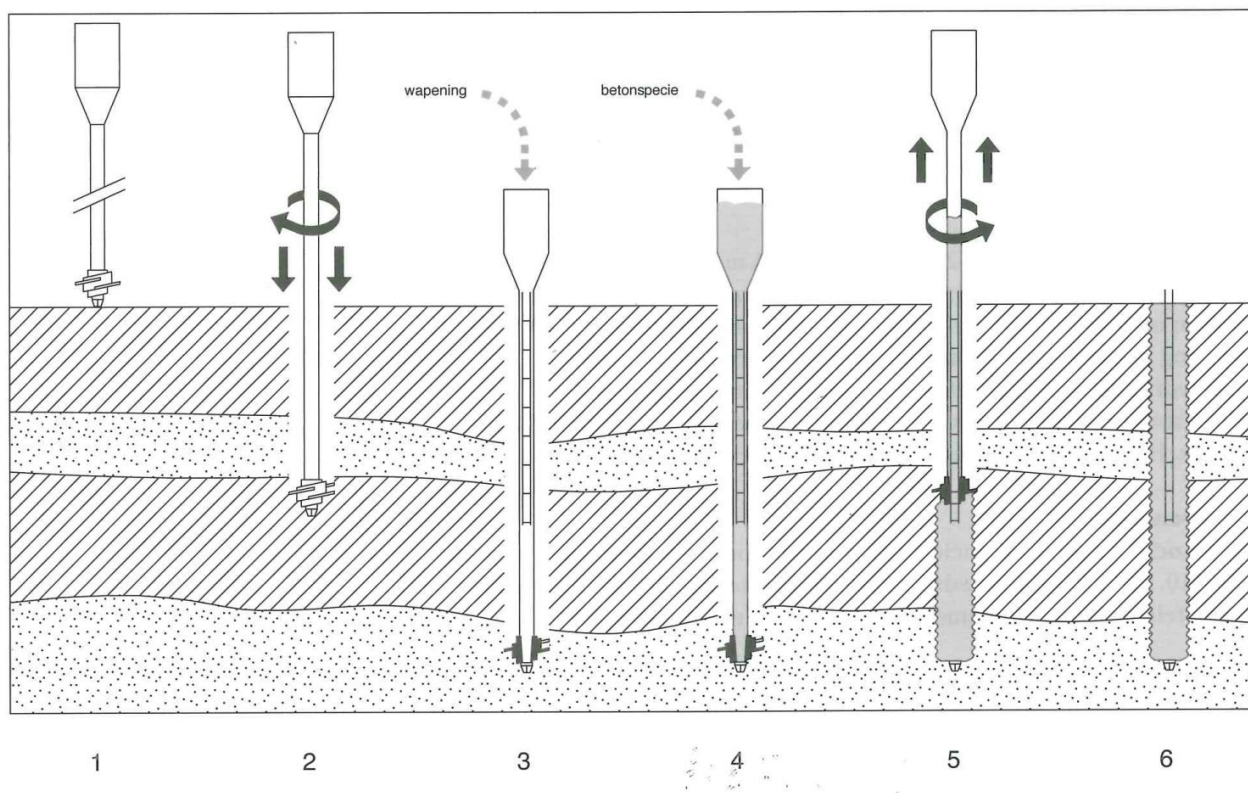
FIGUUR 33 DPA-PLUS INSTALLATIEWIJZE
