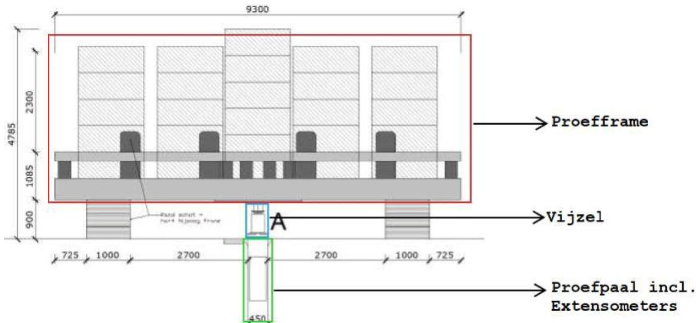
FIGUUR 11 TEKENING VAN DE PROEFPAAL MET VIJZEL OP REACTIEFRAME MET BALLAST
