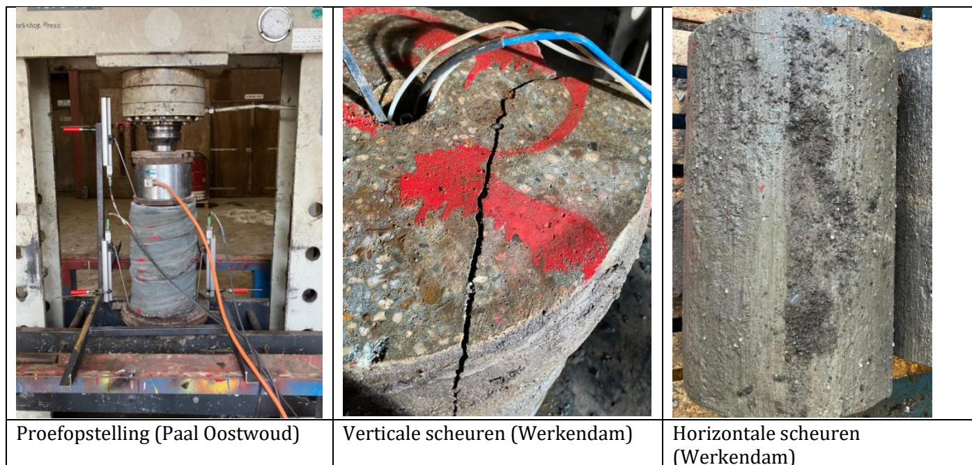
Figuur 28 Opstelling drukbank bij verschillende palen
